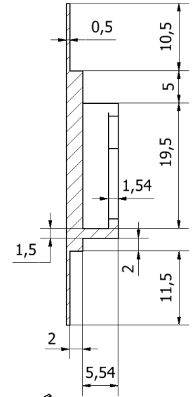
A-A (2 : 1)
