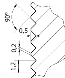
B (8 : 1)
