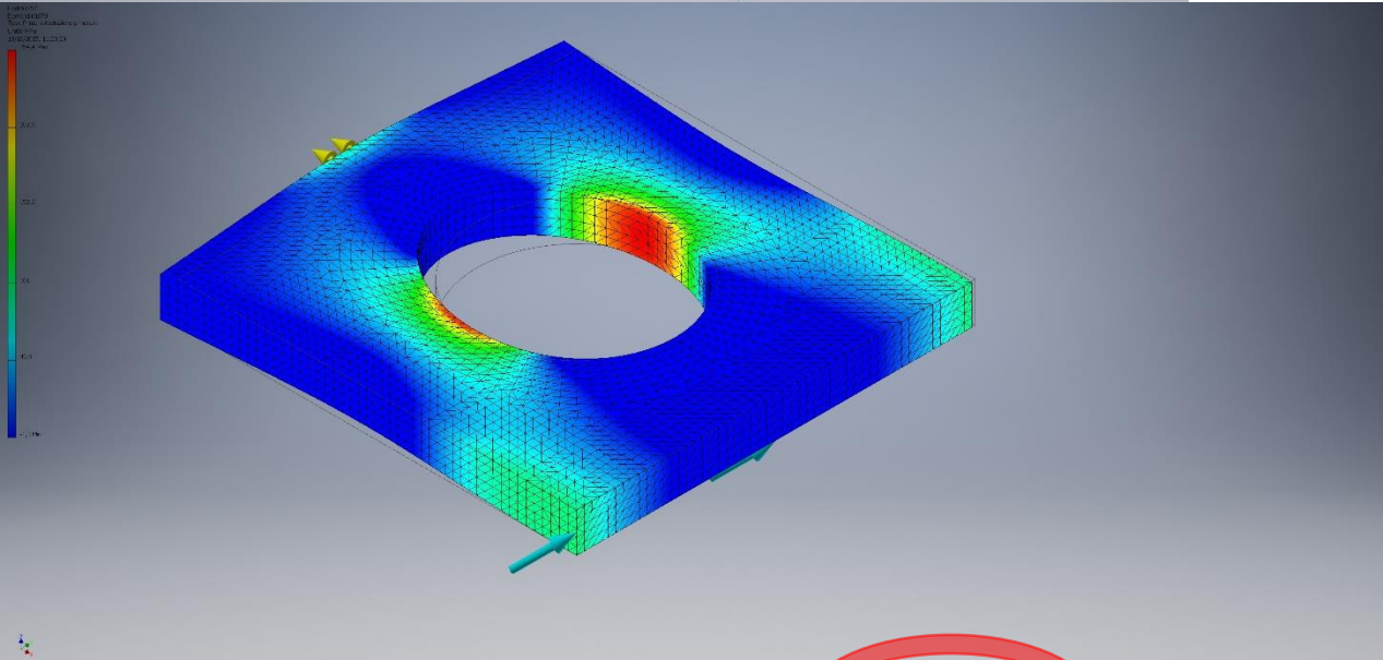
Prima sollecitazione: \sigma_{\text{MAX}} = 254,4 \text{ MPa}
