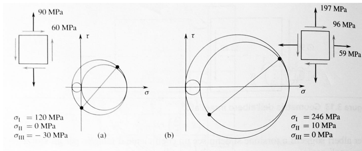
Stato di sforzo agente: (a) albero liscio; (b) albero intagliato.
