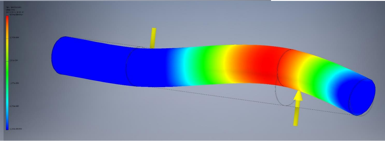
Spostamento: dL_{MAX} = 4,684e-004 \text{ mm}
