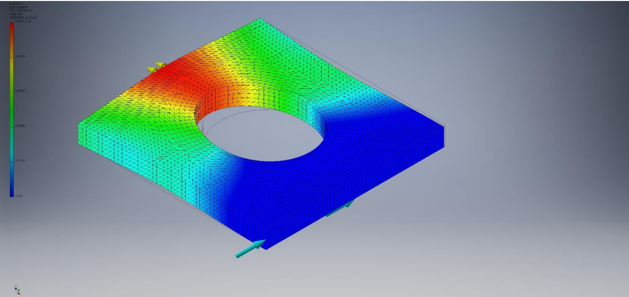
Spostamento: dL_{\text{MAX}} = 0,05012 \text{ mm}
