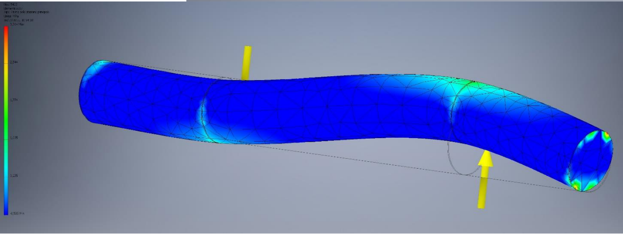
Prima sollecitazione: \sigma_{MAX} = 3,314 \text{ MPa}
