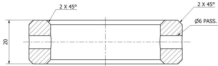
A-A (2 : 1)
